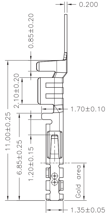
SEC:A-A
