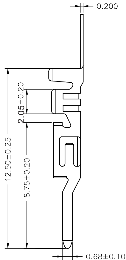
SEC:A-A
