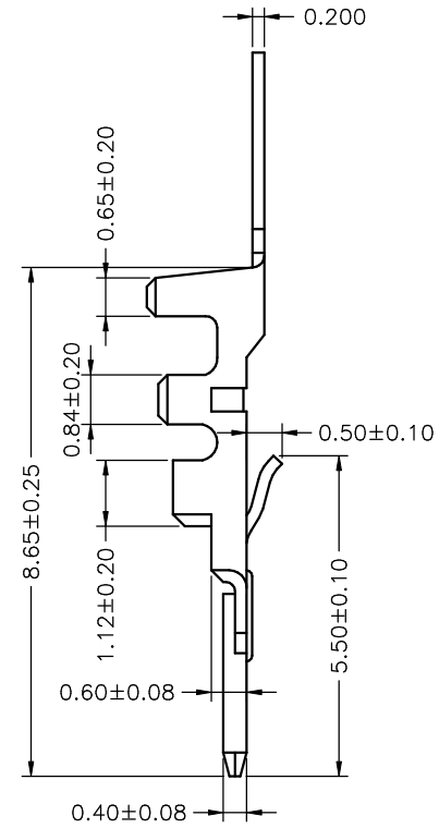
SEC:A-A
