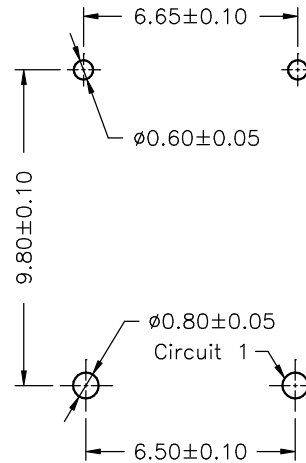
P.C.B LAYOUT
