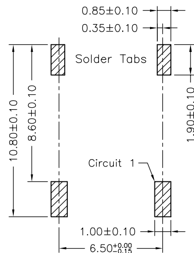
P.C.B LAYOUT
